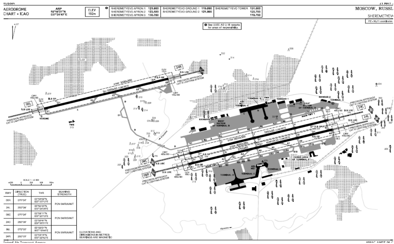
Рисунок 1 – Схема генерального плана международного аэропорта «Шереметьево»
