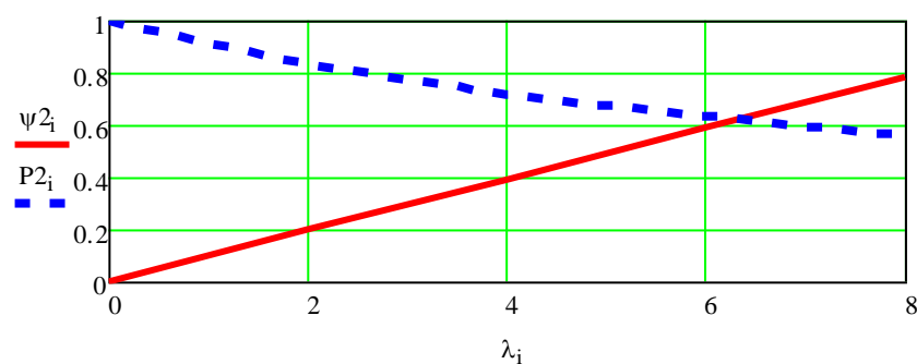
Рис. 2. График загрузки диспетчера \psi_2 и вероятности выполнения операций P_2 от интенсивности потока
