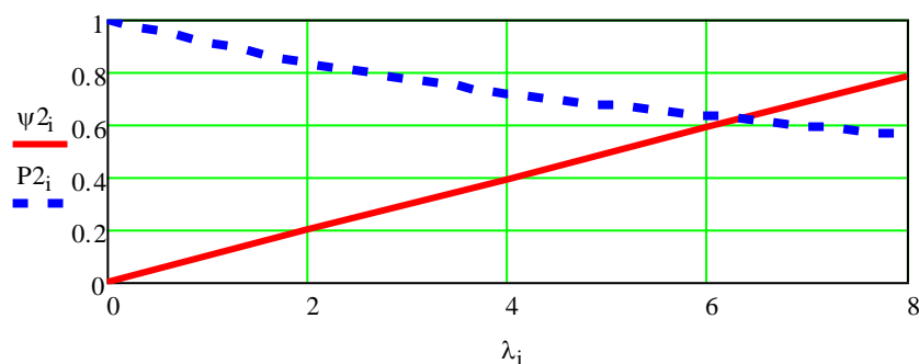
Рис. 2. График загрузки диспетчера \psi_2 и вероятности выполнения операций P_2 от
