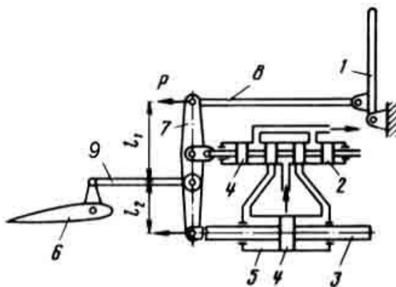
Рисунок 2 - Схема обратимого гидроусилителя: 2 – рычаг управления рулем; 2 – золотник; 3 – шток; 4 – поршень; 5 – гидроцилиндр; 6 – руль; 7 – качалка; 8, 9 - тяги
