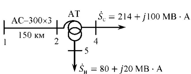
Рис. 2.1. Схема сети
